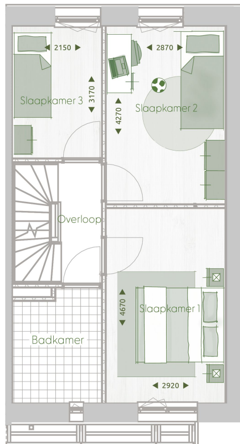
EERSTE VERDIEPING
